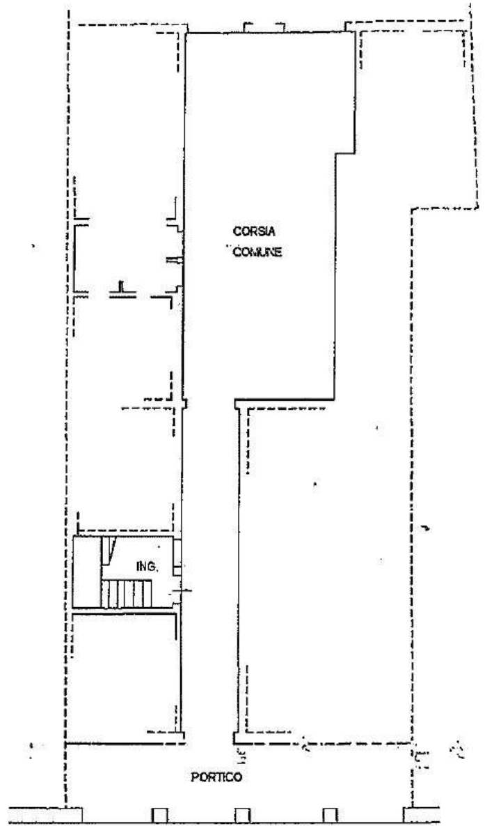
PIANTA PIANO TERRA H cm 275
