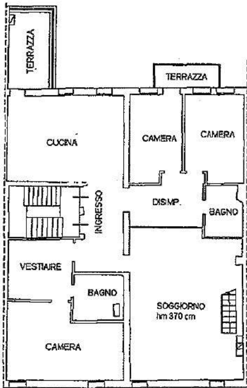
PIANTA PIANO SECONDO H cm 276
